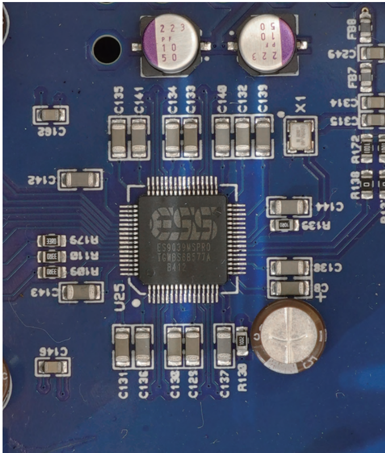
ESS Technology 社の SABRE PRO DAC シリーズのフラッグシップ DAC、ES9039MSPRO を搭載。
