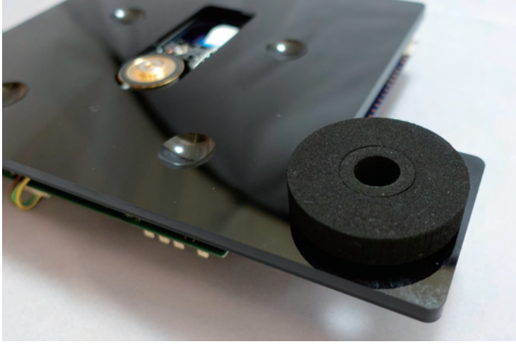
ドライブレカがマウントされたアクリルプレートを硬質スポンジで挟み込みフローティングして搭載
