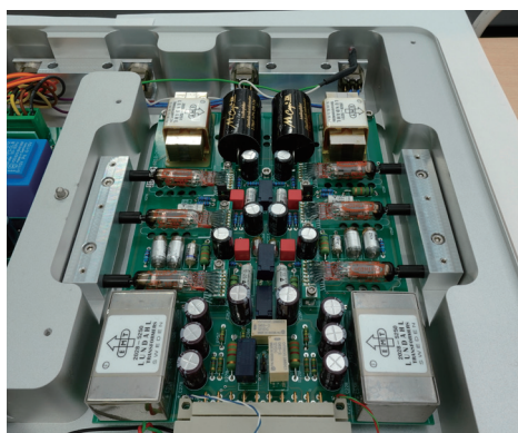
フォノ回路
