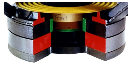
314mm φ SL ウーファー磁気回路
