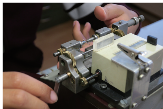
ハンドメイドの精密コイル
